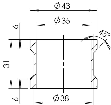
Boccola Cod.206279
